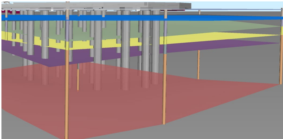
Abb. 3.1.13-1: Praxisbeispiel: Geologisches Schichtmodell mit Homogenbereichen.
