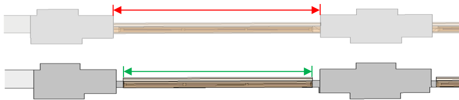
Abb. 3.1.21-4: Interpretationsansätze eines Fensterelements im Grundriss (oben: Fensterrahmen zu breit angenommen, unten: Konstruktiv korrekte Zuordnung).
