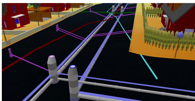
Abb. 3.2.1-4: Unterirdische Leitungsverläufe.
