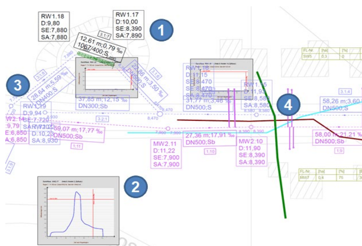
Abb. 3.2.1-2: Ausschnitt Kanallageplan.
